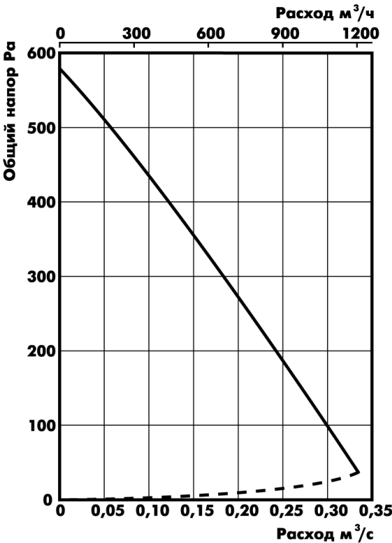
СК 250 С
