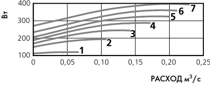
МОЩНОСТЬ/РАСХОД
