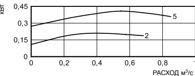
МОЩН./РАСХОД
