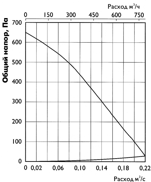
SAU 200 C3
