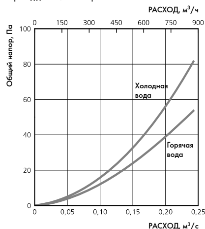
ВОДЯНОЙ НАГРЕВАТЕЛЬ Heru 130 S and 180 S. 5 kW вкл. 2- или 3-ходовой клапан и двигатель клапана, а также датчик против обмораживания.
