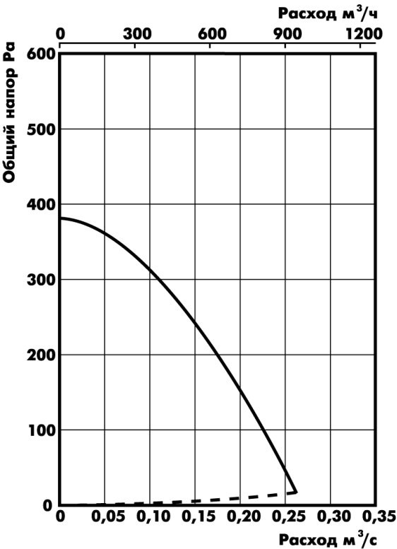
СК 250 А
