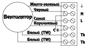
Схема № 6 ~ 220В, 1 фаза, вынесенный термоконт
