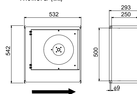
РАЗМЕРЫ (мм)
