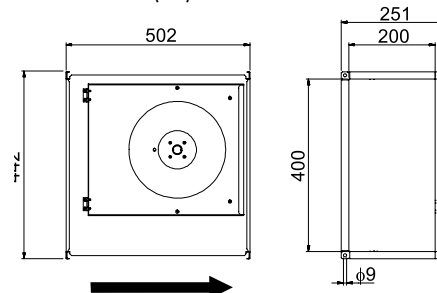
РАЗМЕРЫ (мм)
