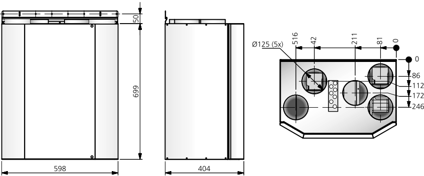
РАЗМЕРЫ (мм)
