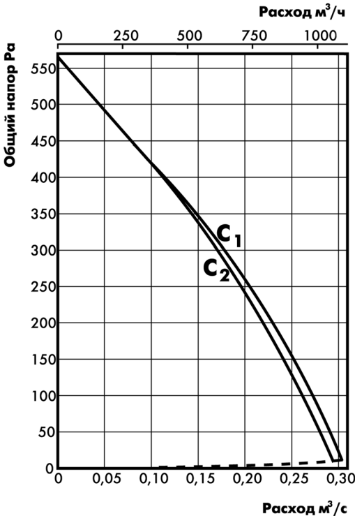
CV/KV 250 C
