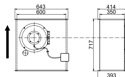
РАЗМЕРЫ (мм)
