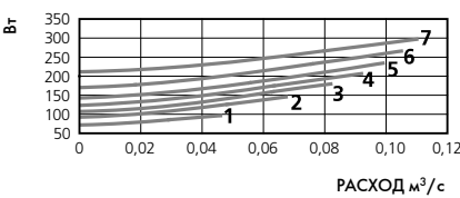
МОЩНОСТЬ/РАСХОД
