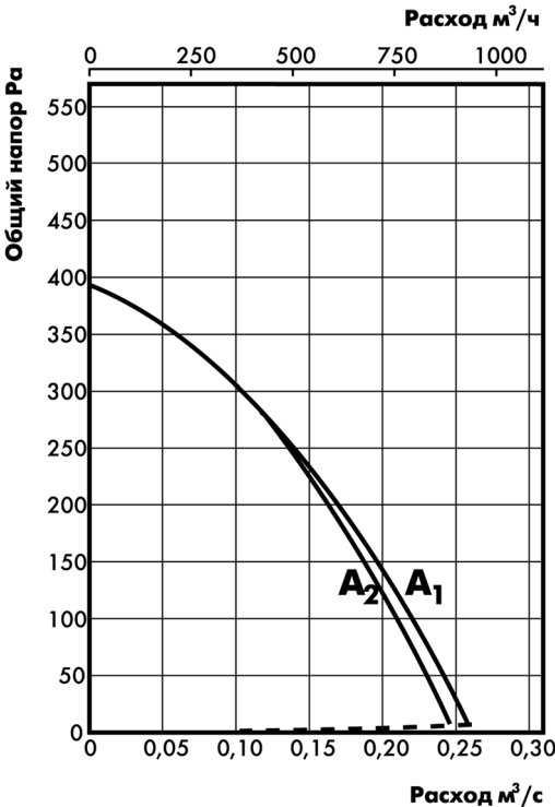
CV/KV 250 A
