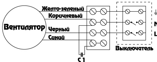
Схема № 11 ~ 220В, 1 фаза, внешний выключатель
