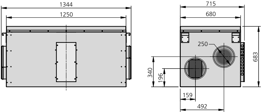
РАЗМЕРЫ (мм)
