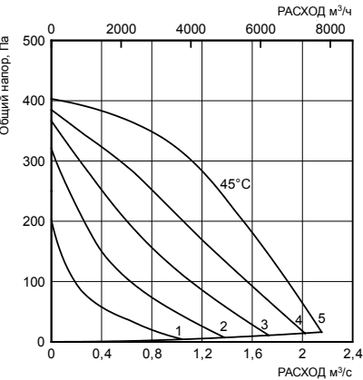
НАПОР/РАСХОД
